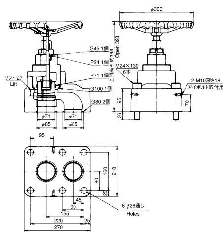
HG-4211-80-23 質量 Mass :52.3kg
