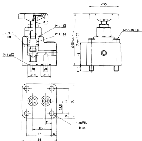
HG-4211-8-34 質量 Mass :1.4kg
